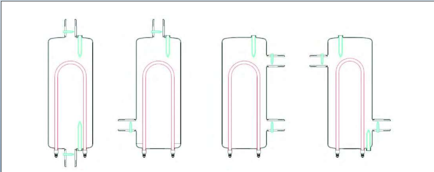
红色的是铠装式管状加热器。蓝色的是：温度传感器探温棒热电偶套管
