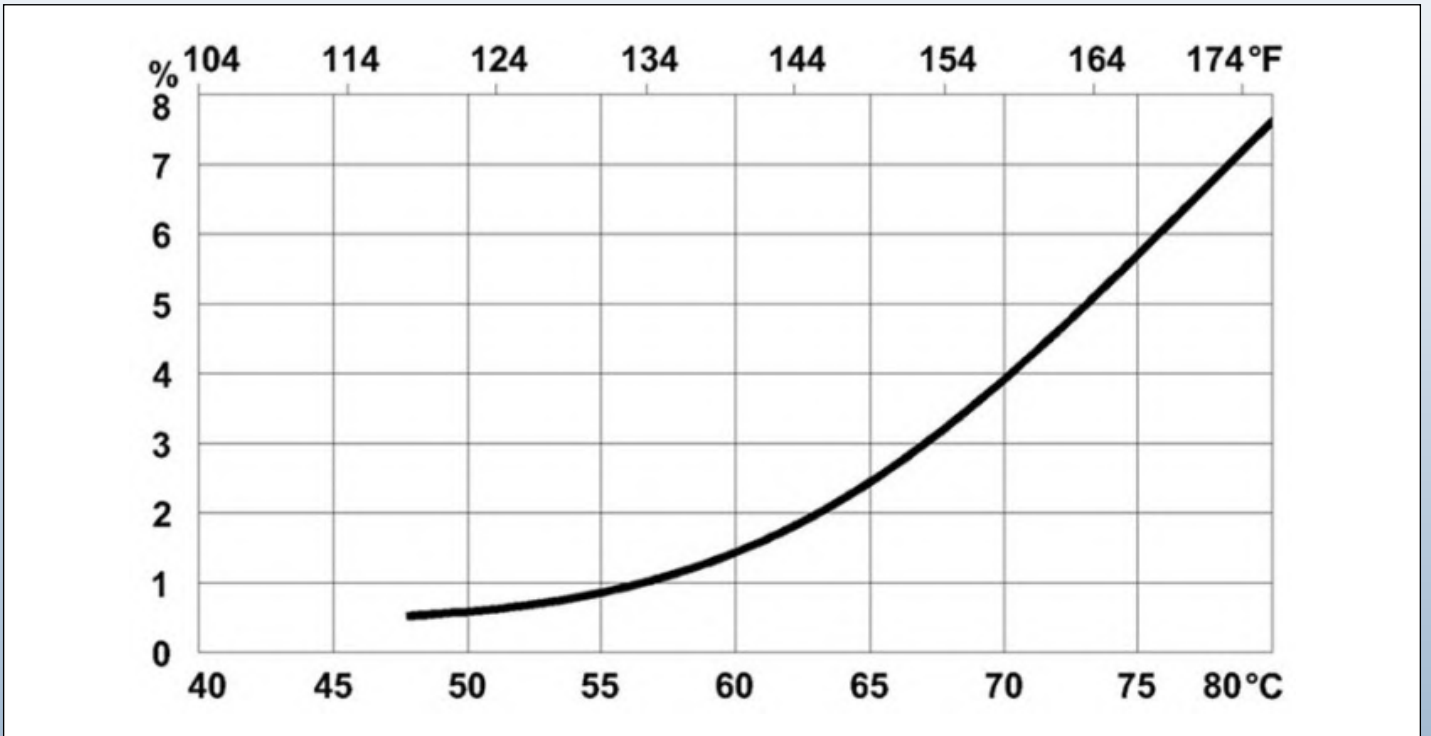
K-2 水垢沉淀与温度的对比
